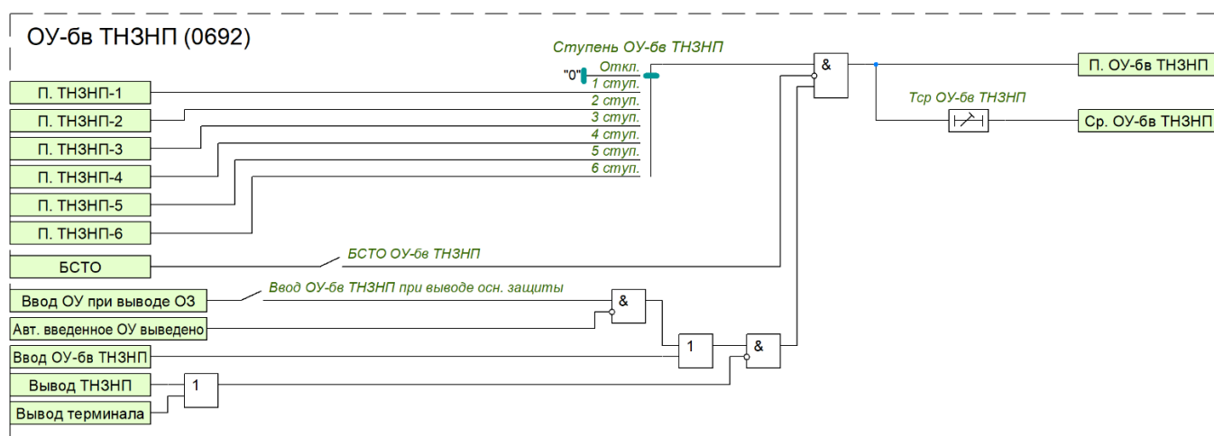
Рисунок 1.23 – Функциональная схема ОУ-бв THЗНП
