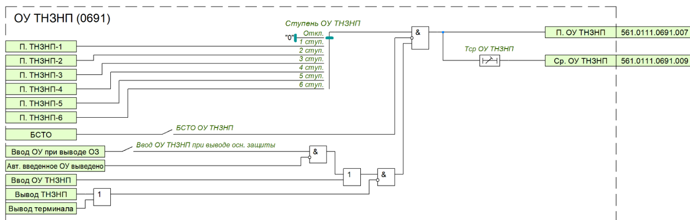
Рисунок 1.22 – Функциональная схема ОУ THЗНП
